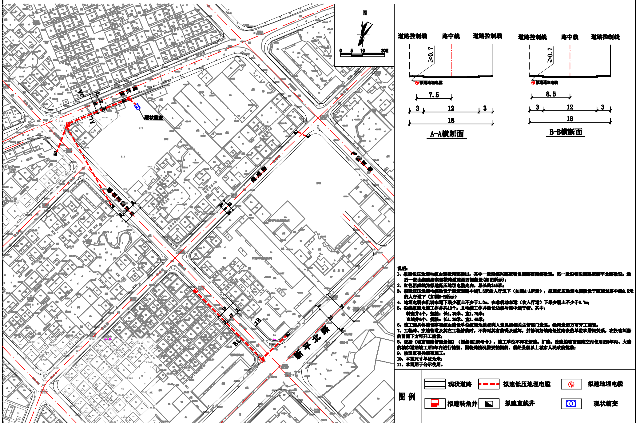
恩平供电局恩城供电所集成公用台变改造工程走向示意图
