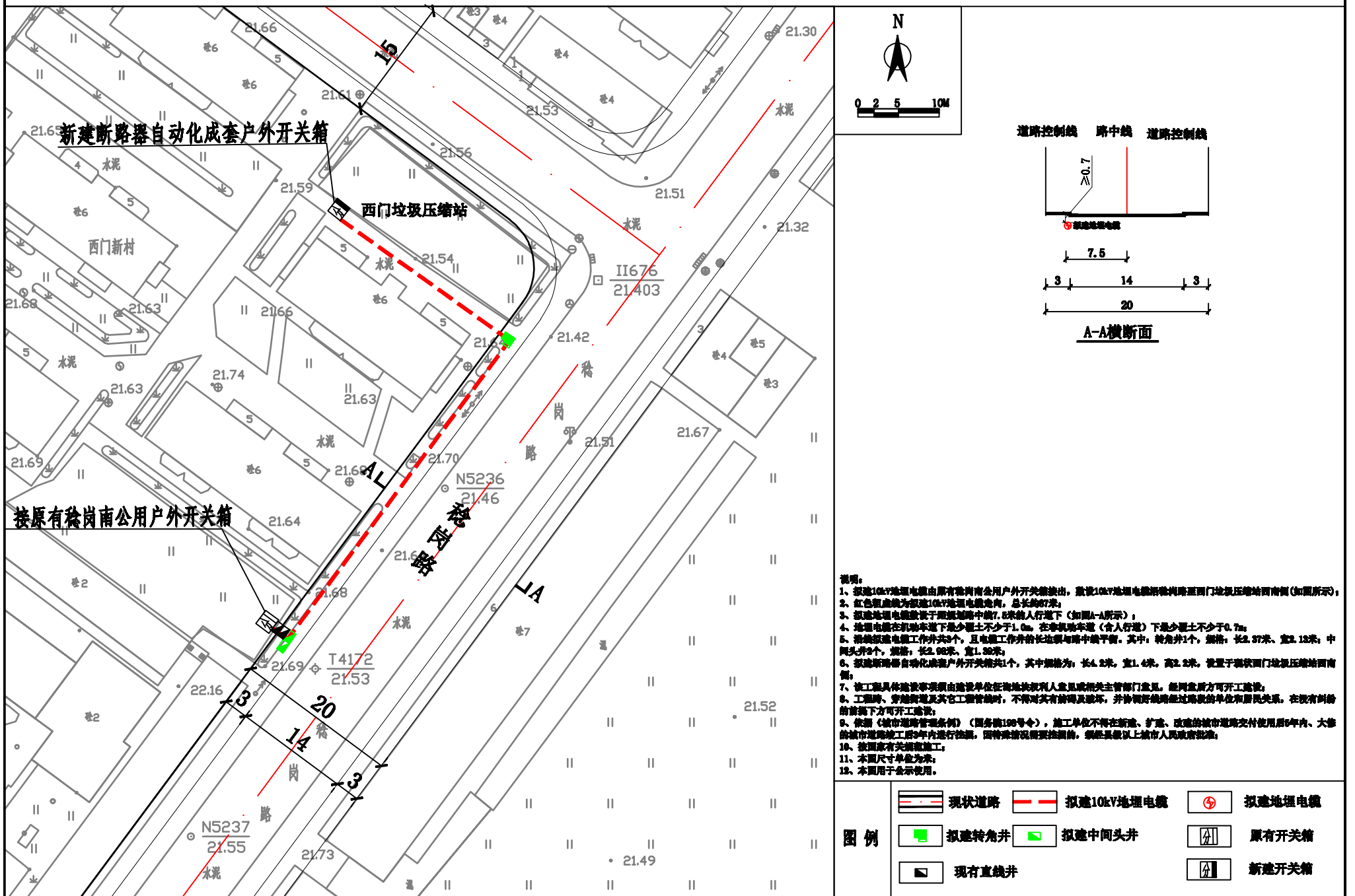
恩平供电局10kV恩金线自动化改造工程走向示意图
