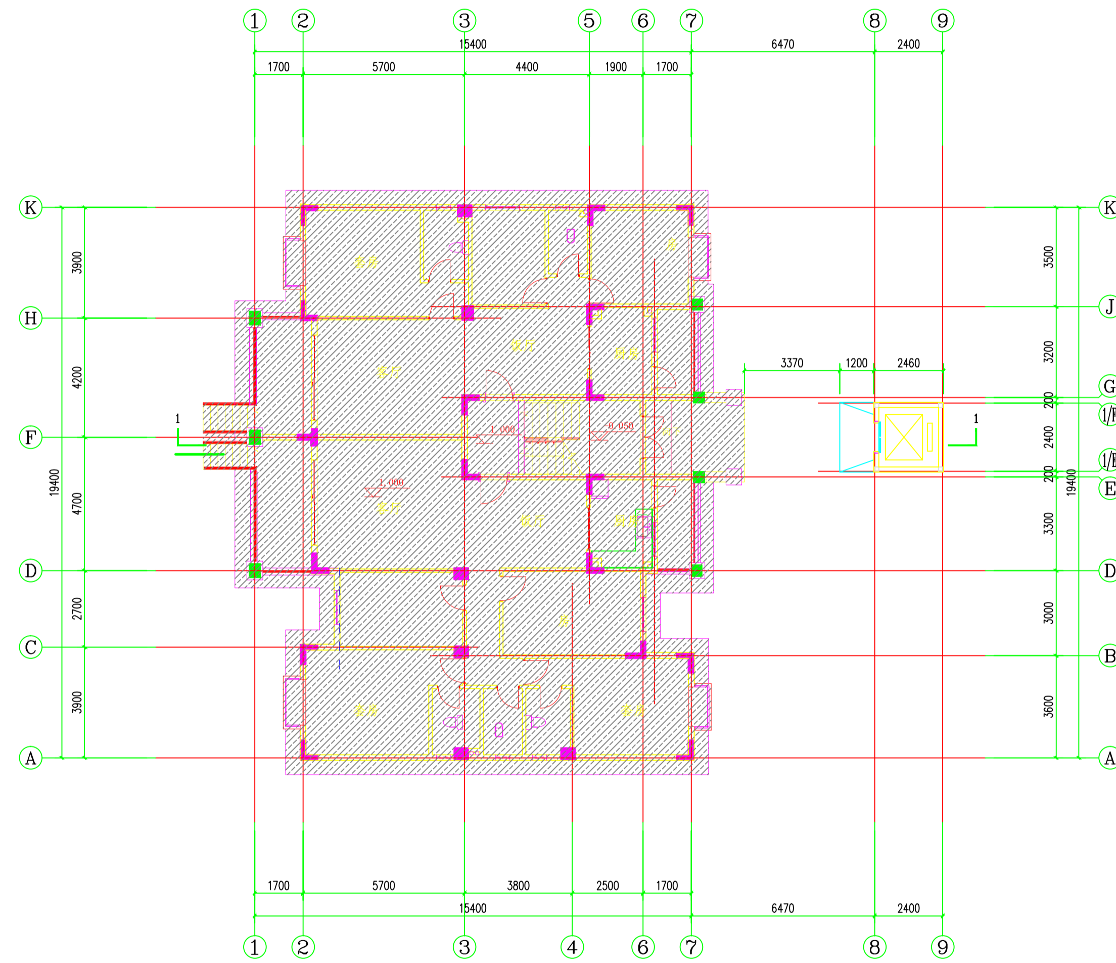
首层平面图 1:100
