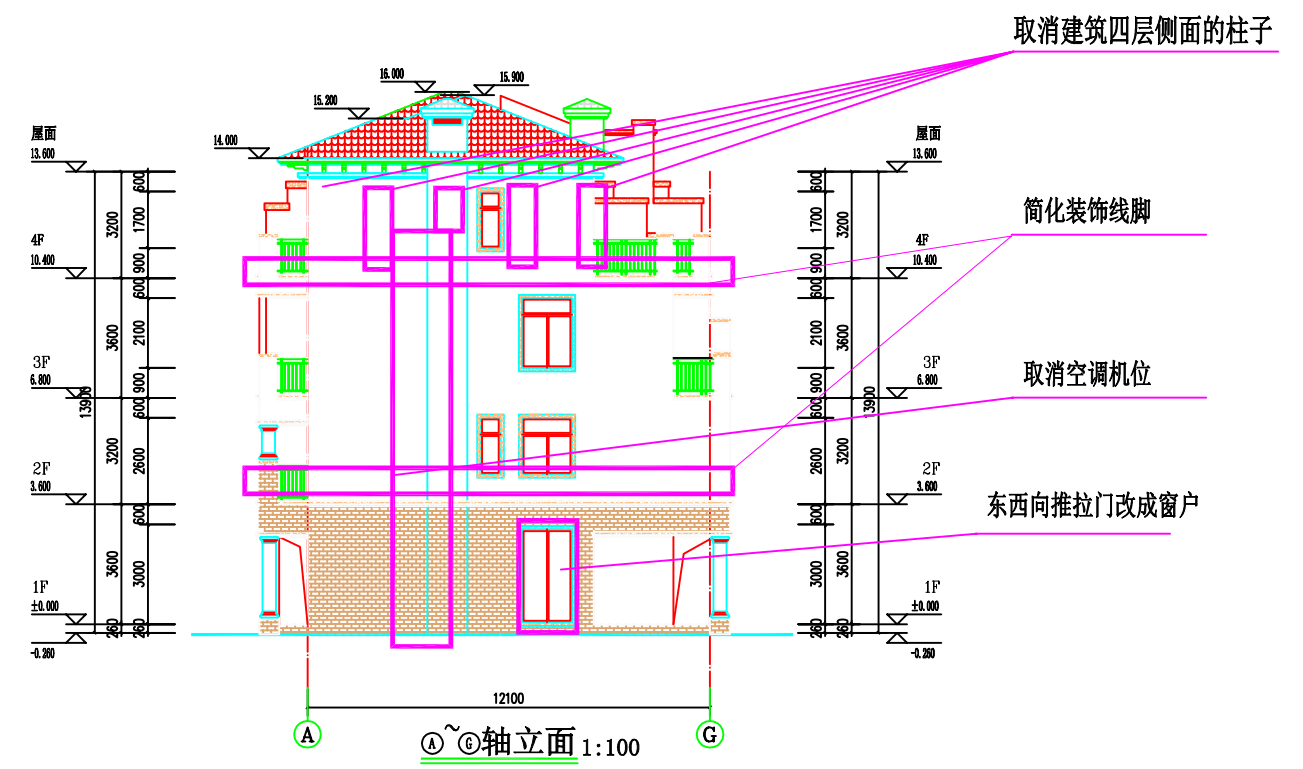
44栋、45栋调整后东立面
