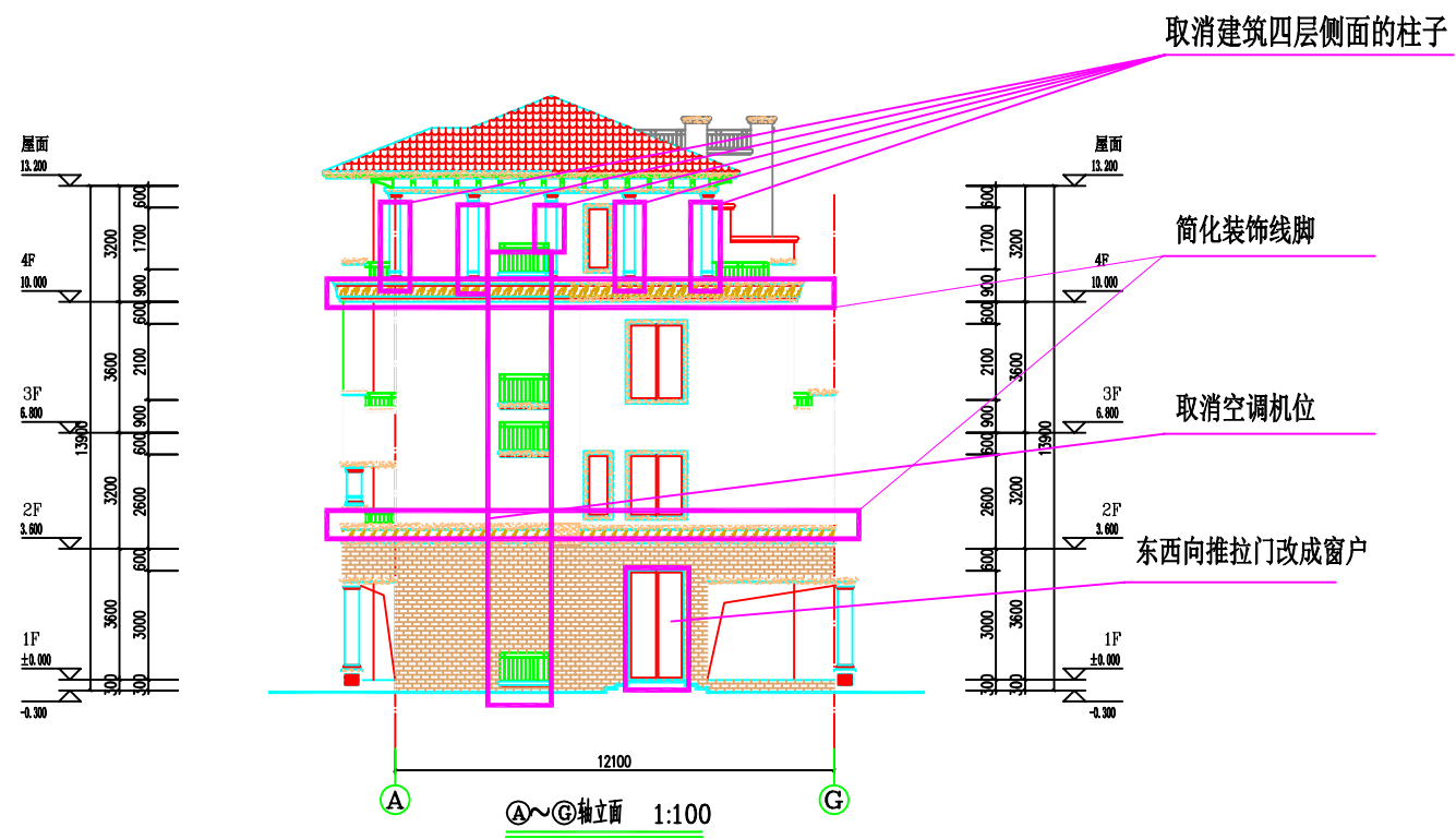
44栋、45栋调整前东立面
