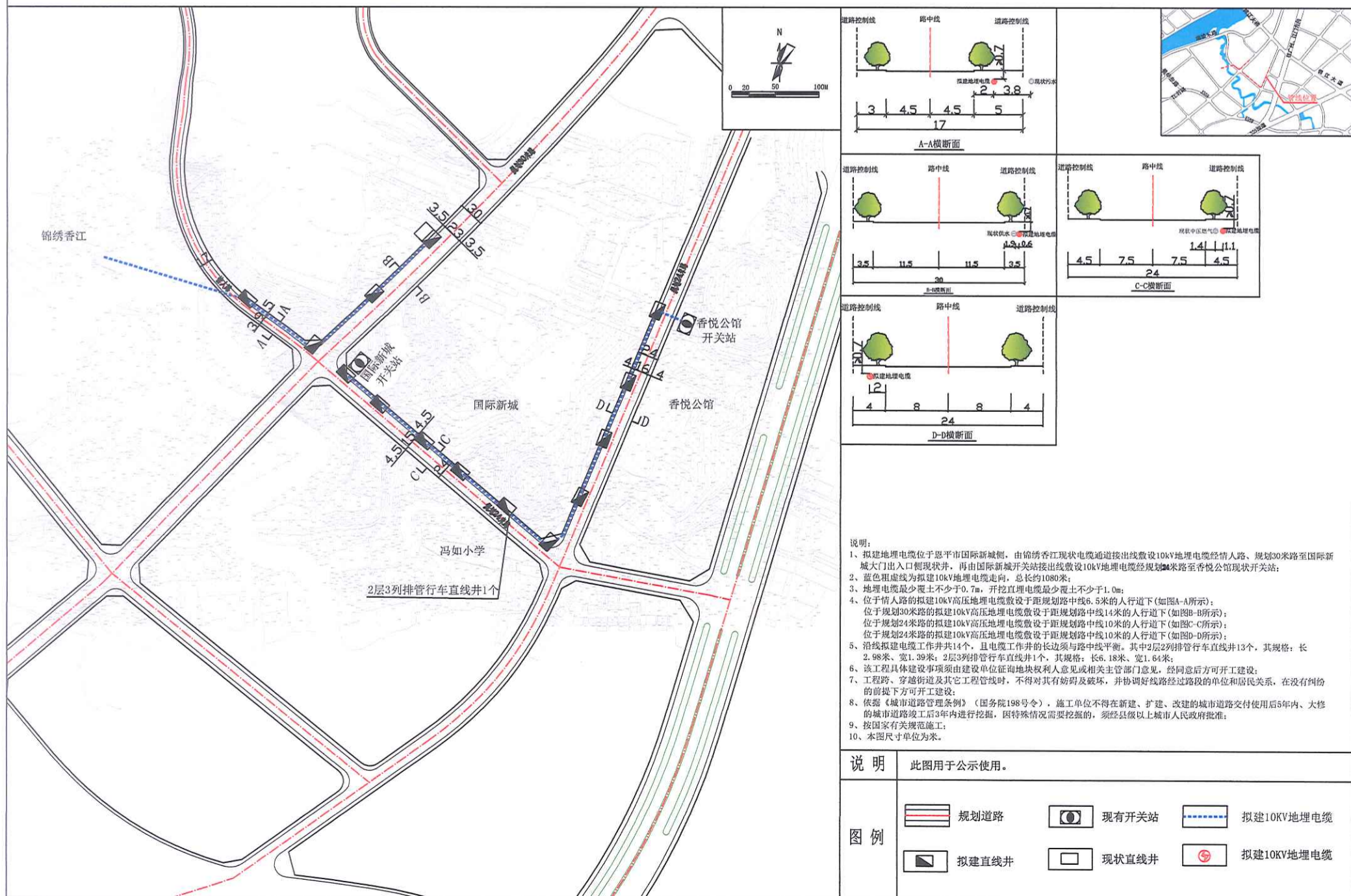
恩平供电局10kV锦绣线、锦新甲线网架完善工程走向示意图（调整方案）
