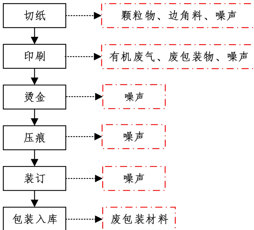
图2 项目纸制品印刷生产工艺流程及产污过程图
