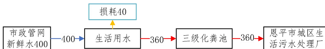
图1 项目后的项目水平衡图(单位 m^3/a )
