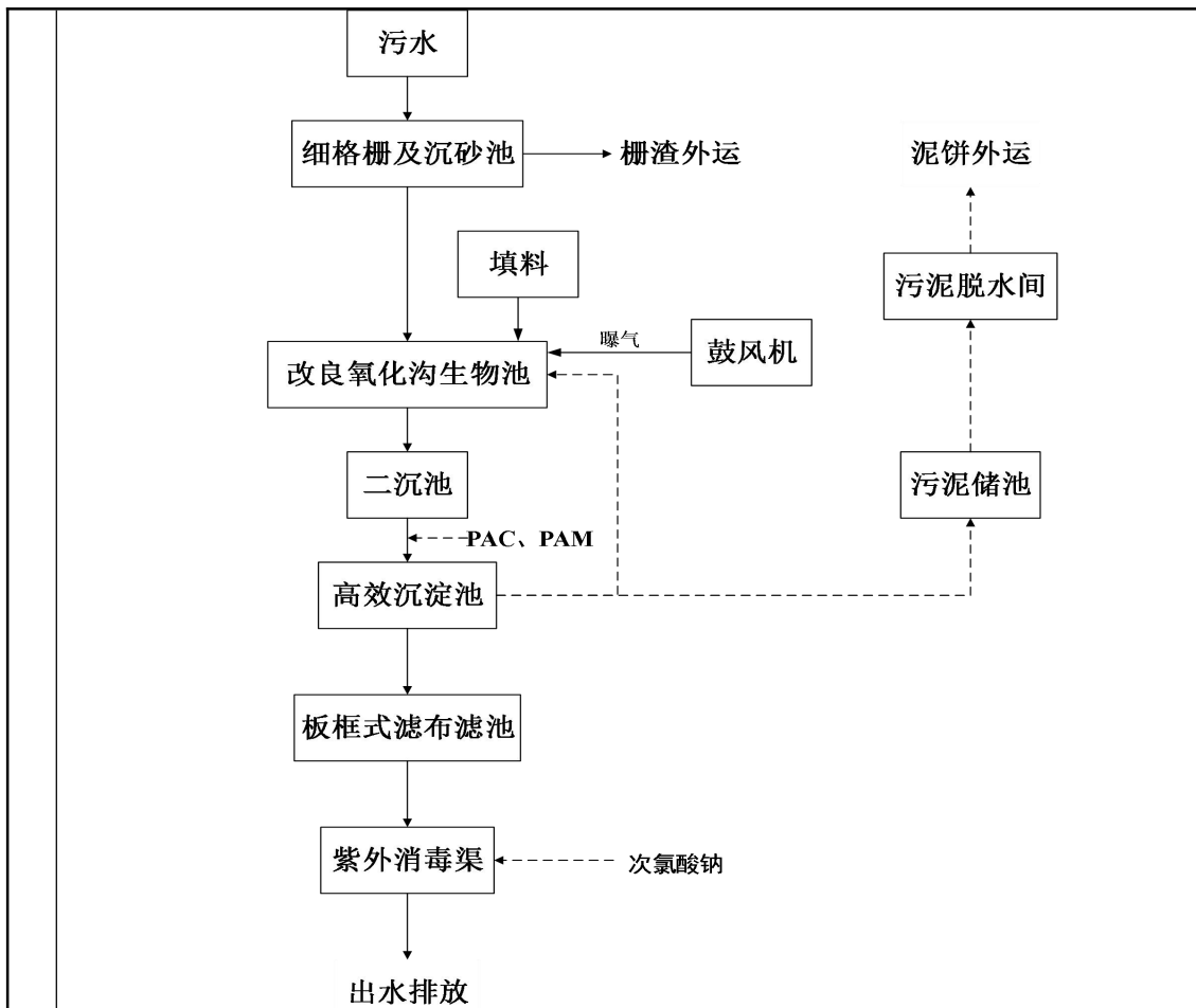
图4 恩平市城区生活污水处理厂工艺流程图
